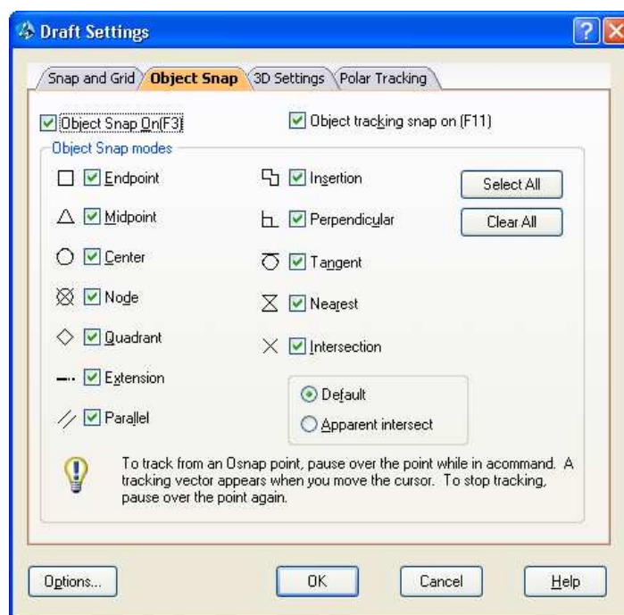
Rys. 9 – Ustawienia rysunku.
